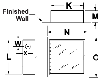
TRIMLESS
