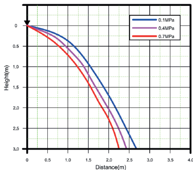
Pendant (LF420/LF421)
